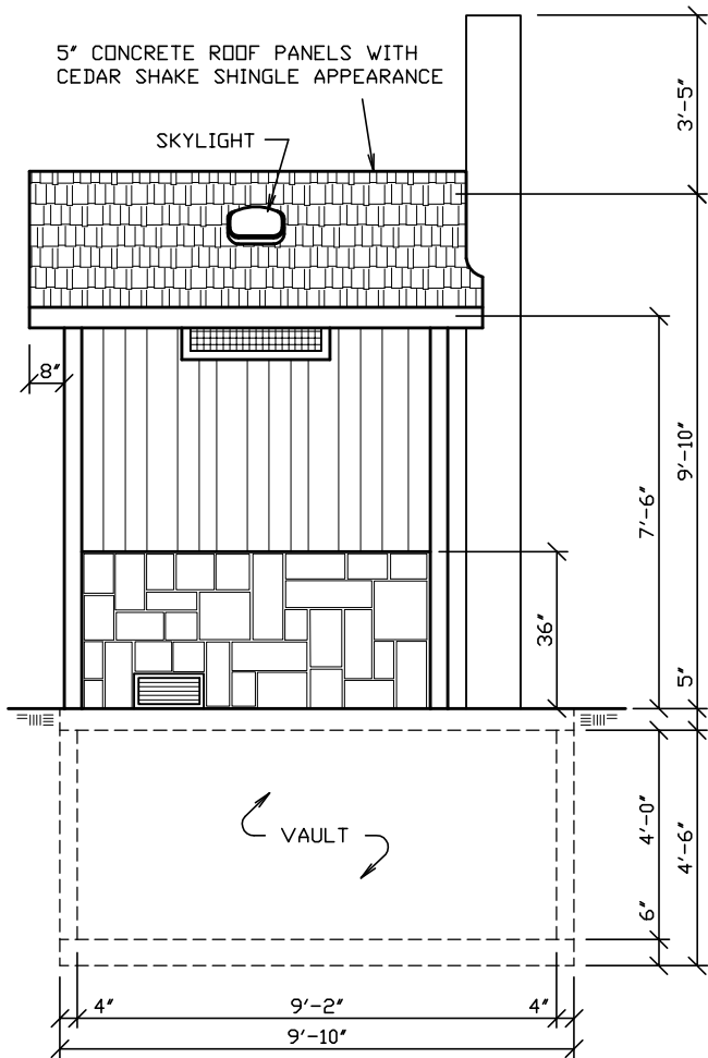
RIGHT ELEVATION SCALE: 1/4" = 1'-0"
