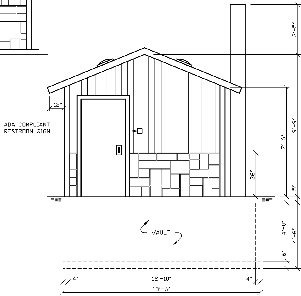
RIGHT ELEVATION SCALE: 1/4" = 1'-0"
