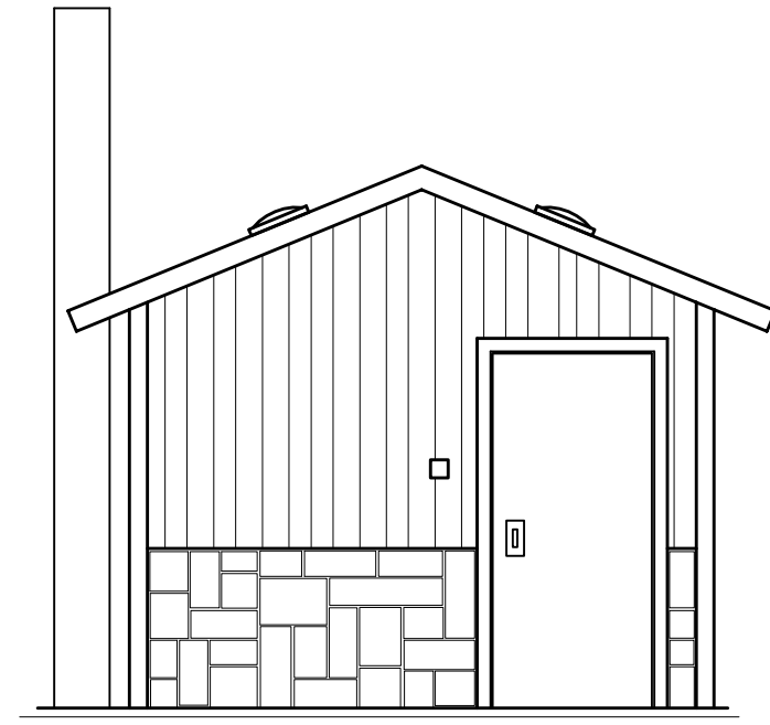
LEFT ELEVATION SCALE: 1/4" = 1'-0"
